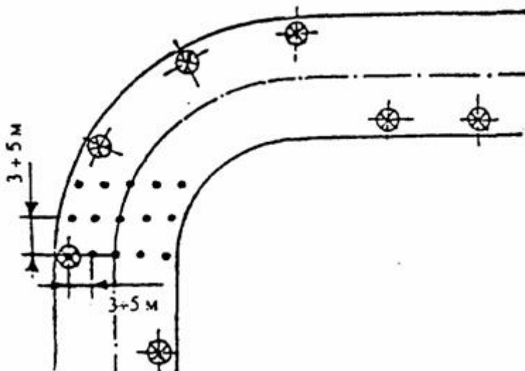
Рисунок А9 — Расположение контрольных точек при измерении средней освещенности улиц на перекрестке
