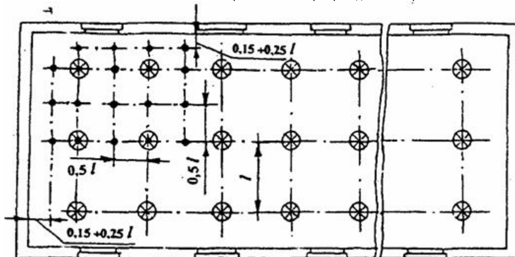
Расположение контрольных точек при проведении измерений
