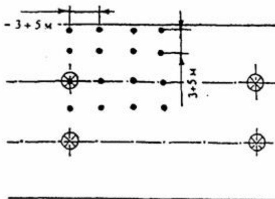
Рисунок А8 — Расположение контрольных точек при измерении средней освещенности улиц при осевом двухрядном расположении светильников
