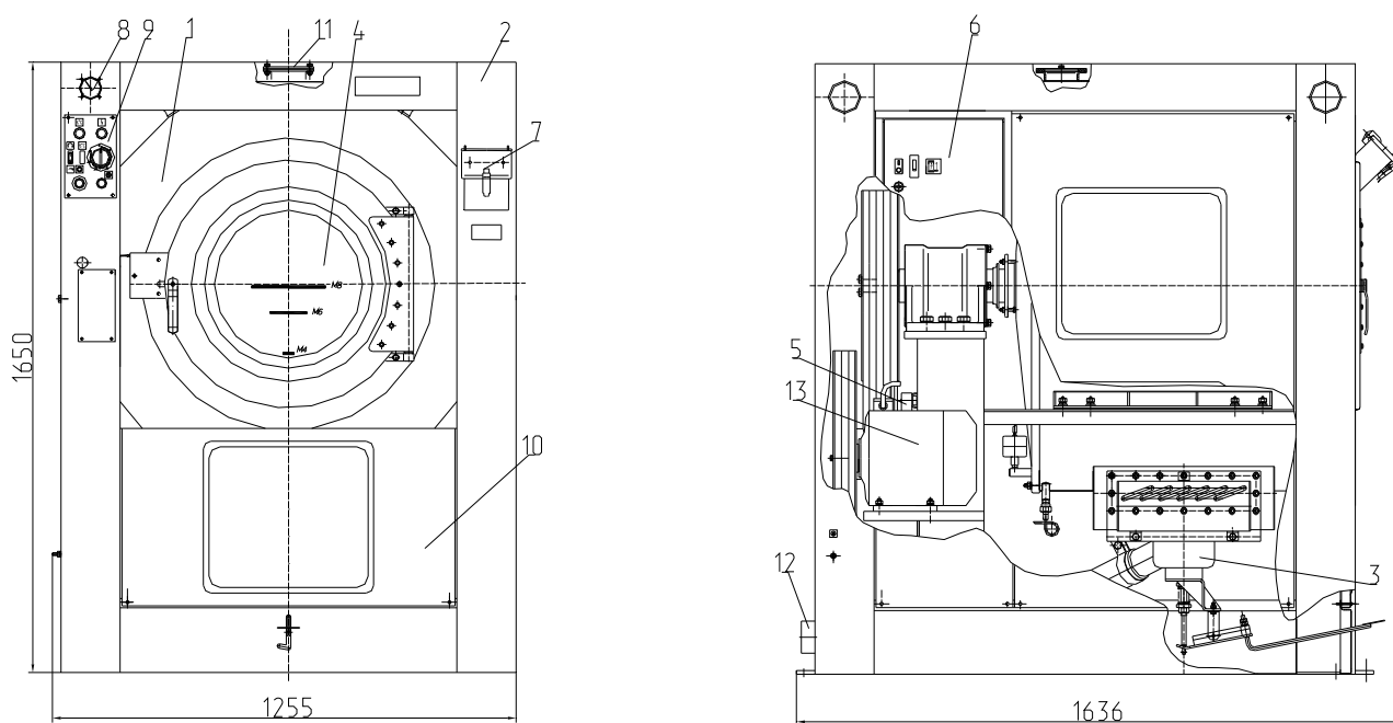
Рис1 Общий вид.
