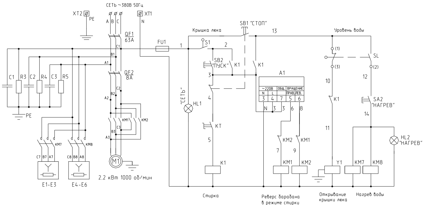
Рис.3а. Схема электрическая принципиальная машины стиральной Л60-121
