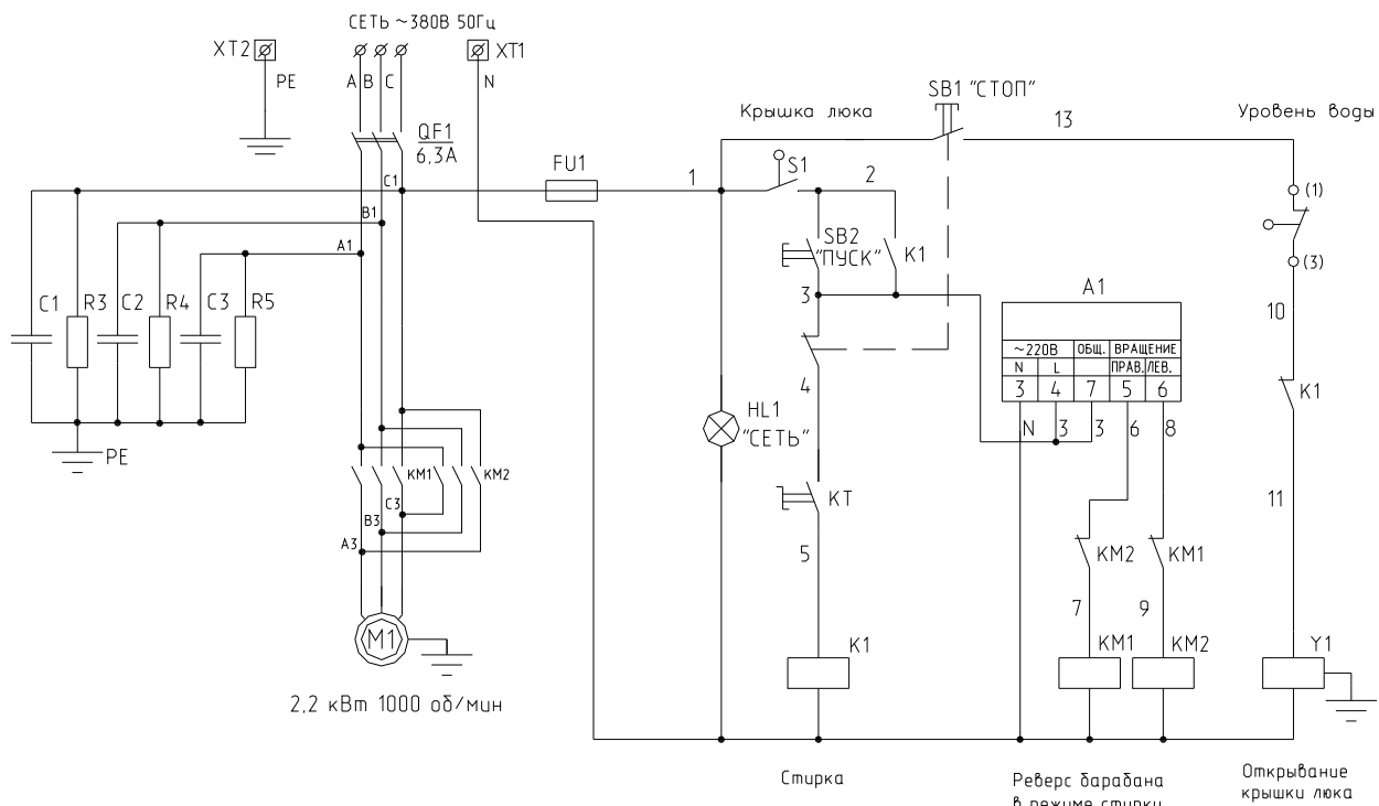
Рис.3д. Схема электрическая принципиальная машины стиральной Л60-111
