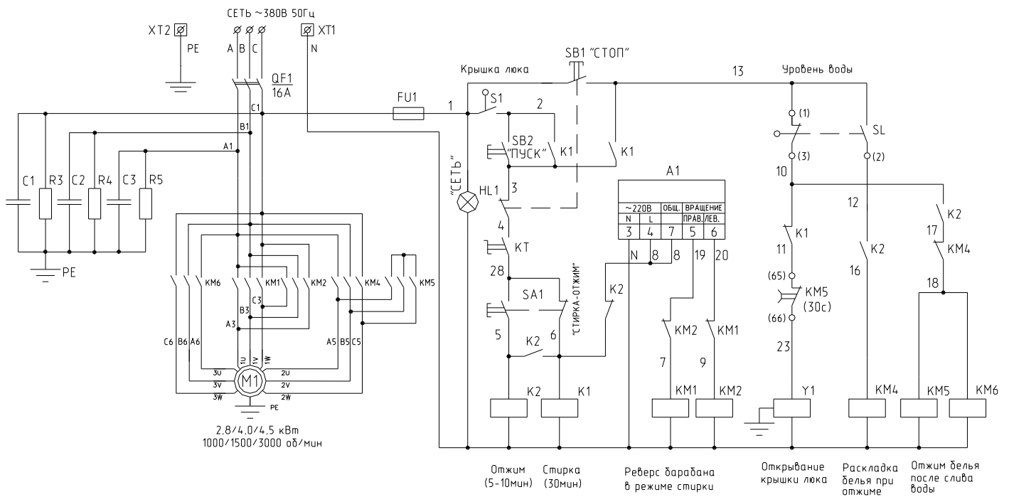
Рис.3з. Схема электрическая принципиальная машины стиральной Л60-211
