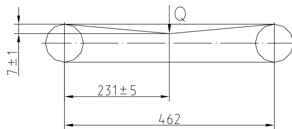
Схема натяжения ремней внутреннего барабана
