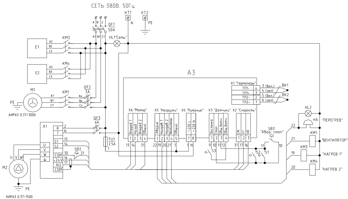
Рис. 3б. Схема электрическая принципиальная каландра гладильного ЛК1840 с вентилятором
