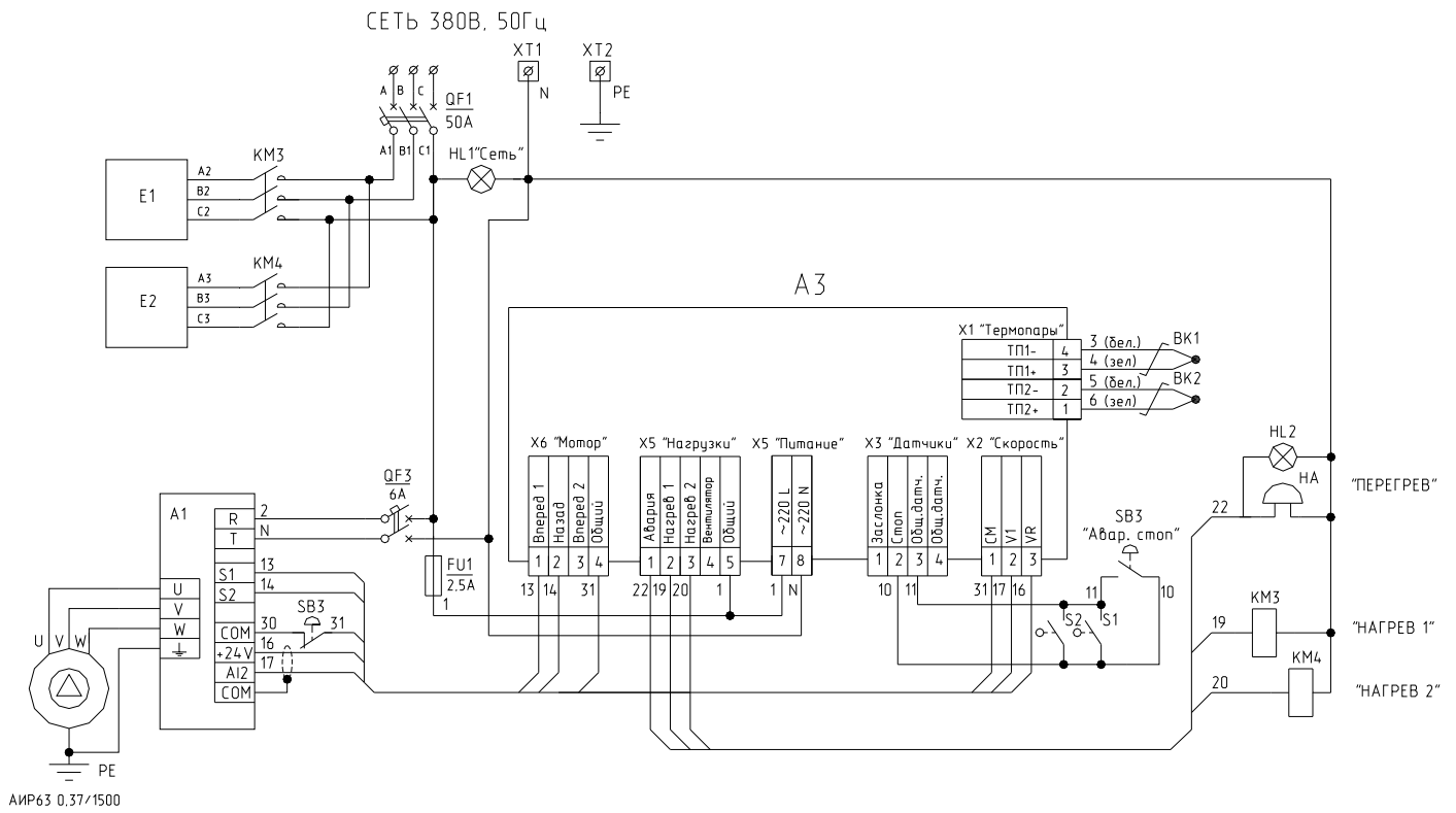
Рис. 3г. Схема электрическая принципиальная каландра гладильного ЛК1840 без вентилятора
