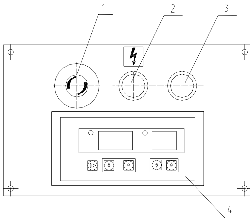
Рис. 5. Расположение органов управления каландра гладильного ЛК1840
