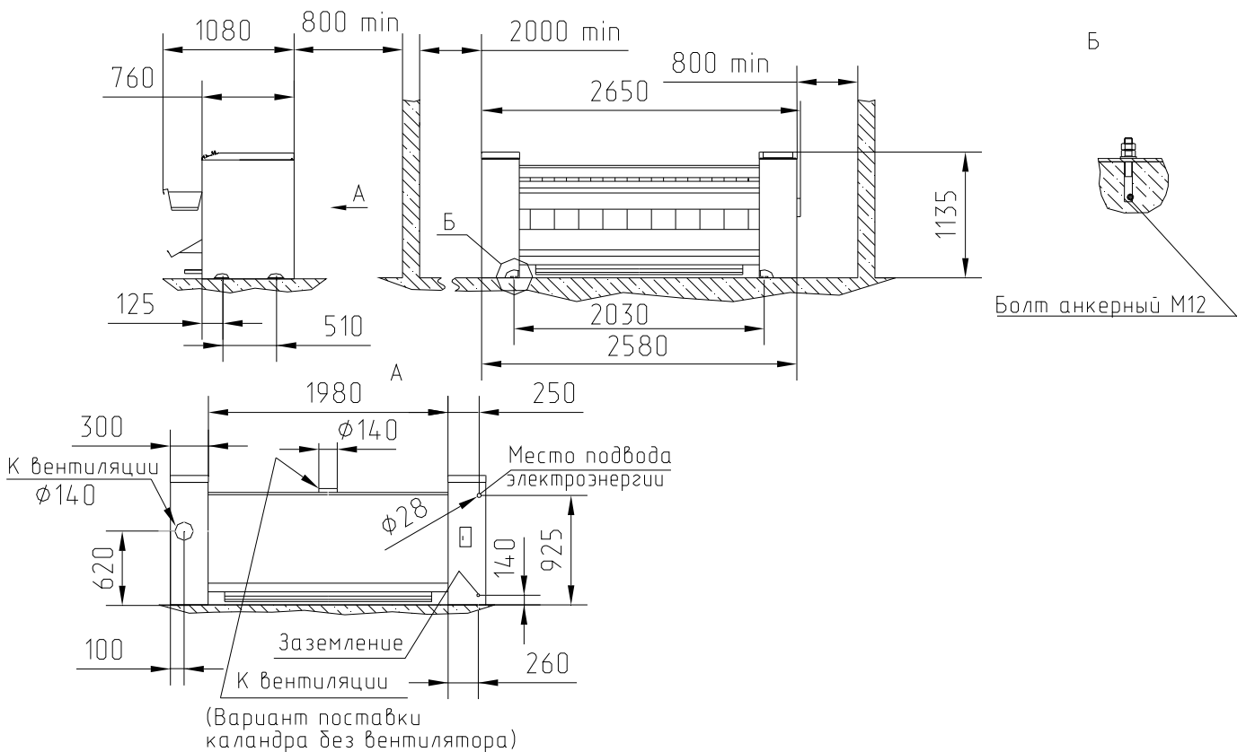
Рис. 7. Монтажный чертеж
