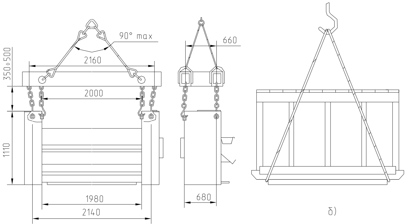
а) Рис.12 Схема строповки каландра а) без тары; б) в таре
