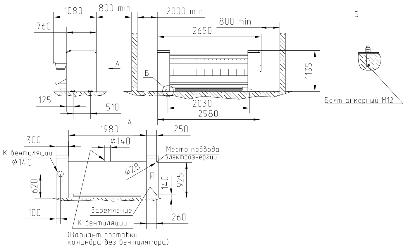
Рис. 7. Монтажный чертеж
