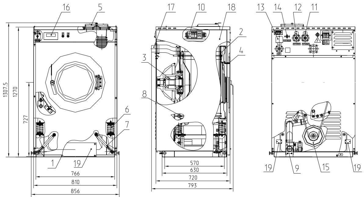
Рис.1 Общий вид
