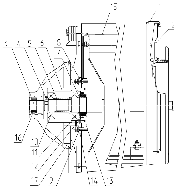
Рис.5 Демонтаж опоры внутреннего барабана
