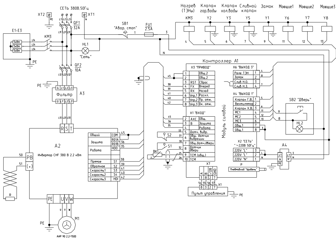
Рис.6а. Схема электрическая принципиальная машины стиральной 10-10 с электрическим обогревом
