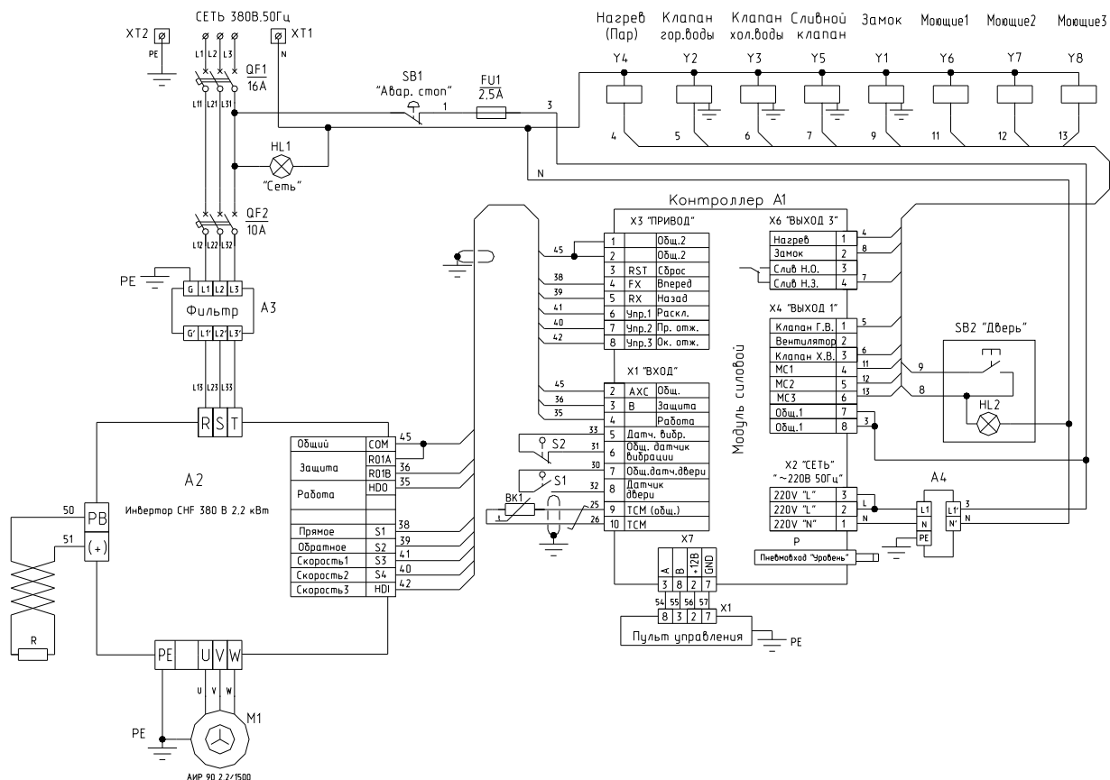
Рис.6б. Схема электрическая принципиальная машины стиральной ЛО-10 с паровым обогревом
