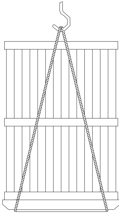
Рис.8. Схема транспортировки
