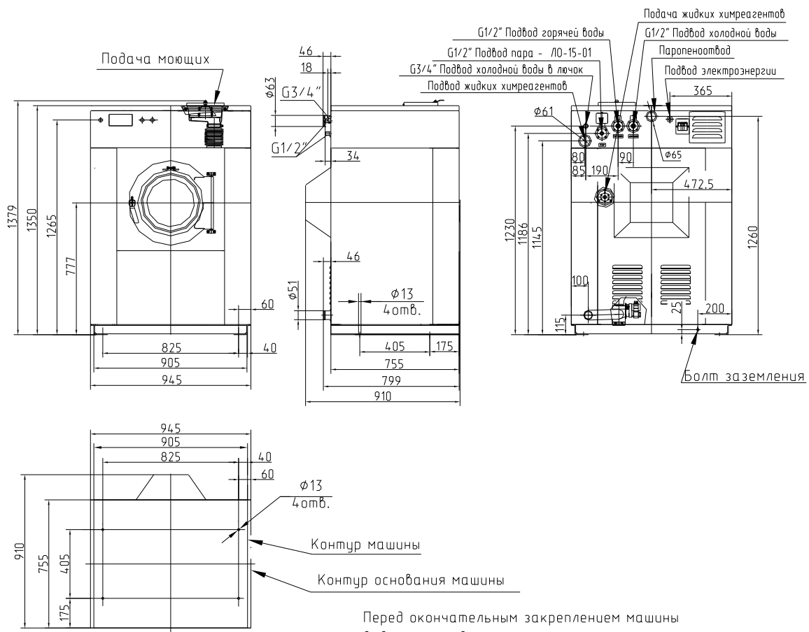
Рис.3 Монтажный чертеж
