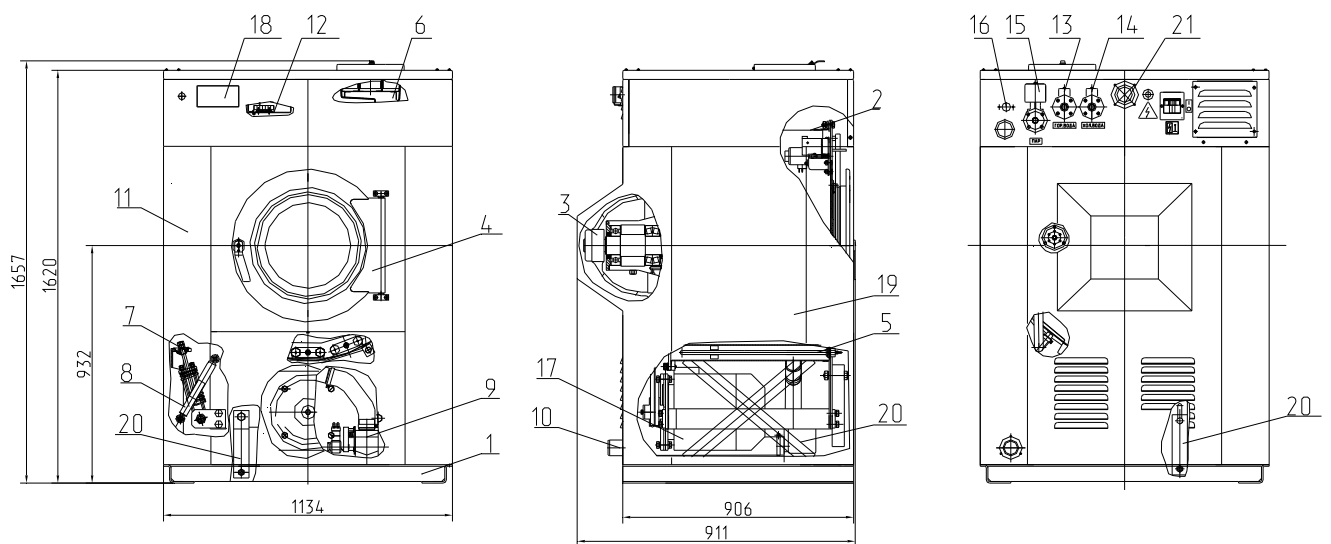
Рис.1 Общий вид
