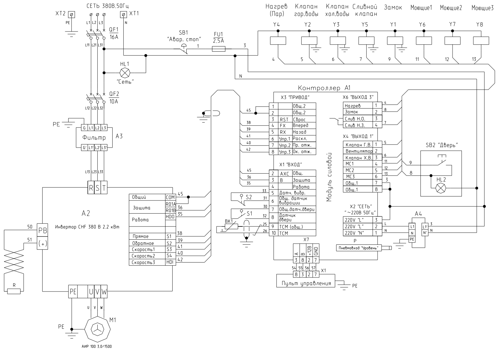
Рис.6б. Схема электрическая принципиальная машины стиральной 10-15 с паровым обогревом
