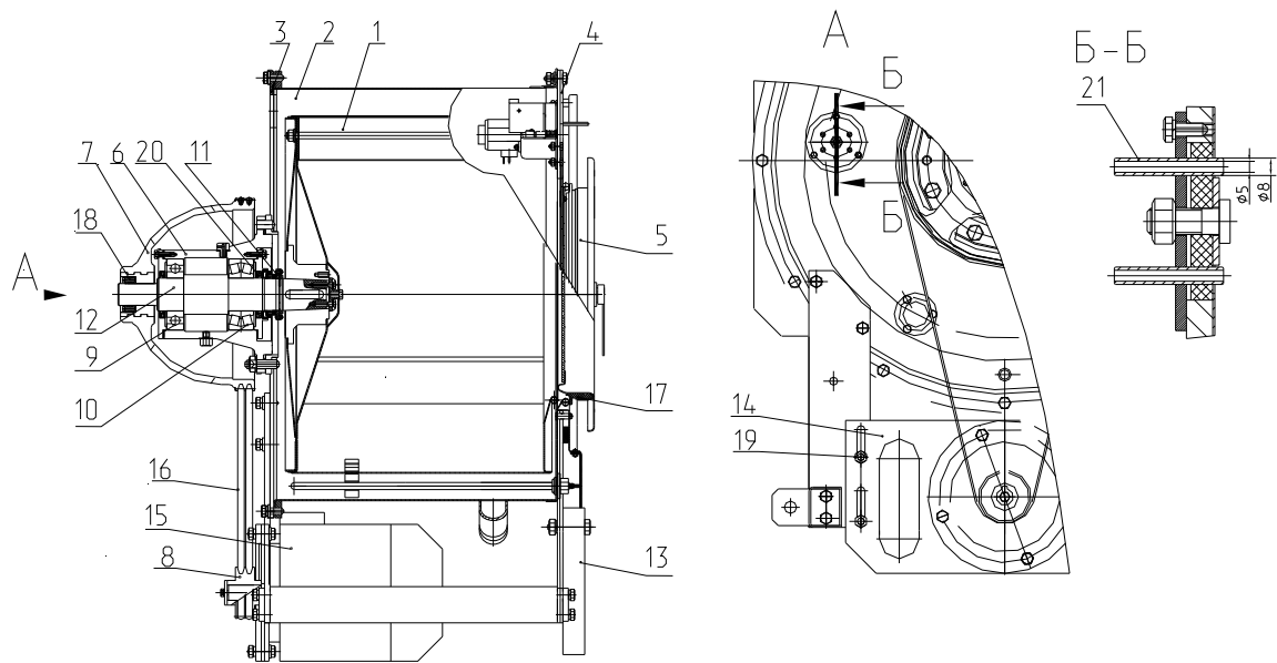
Рис.4 Блок барабанов
