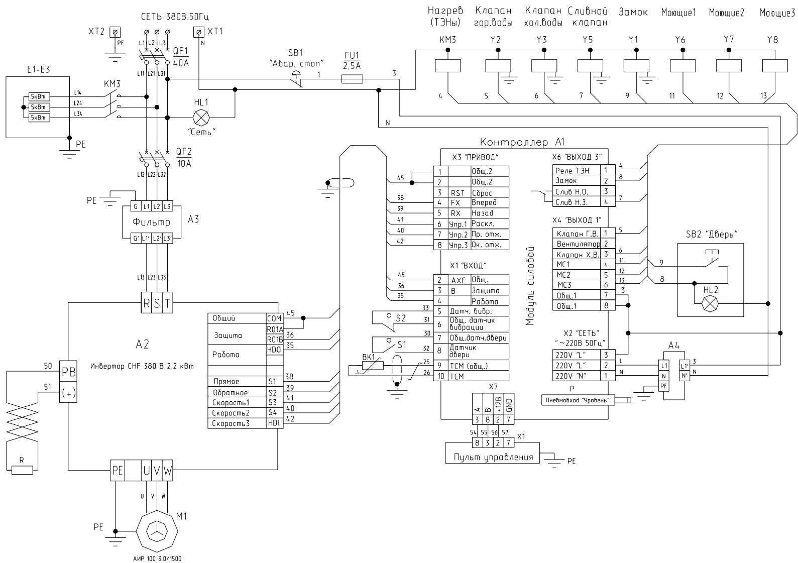
Рис.6а. Схема электрическая принципиальная машины стиральной ЛО-15 с электрическим обогревом
