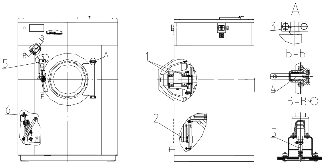
Рис.7 Схема смазки
