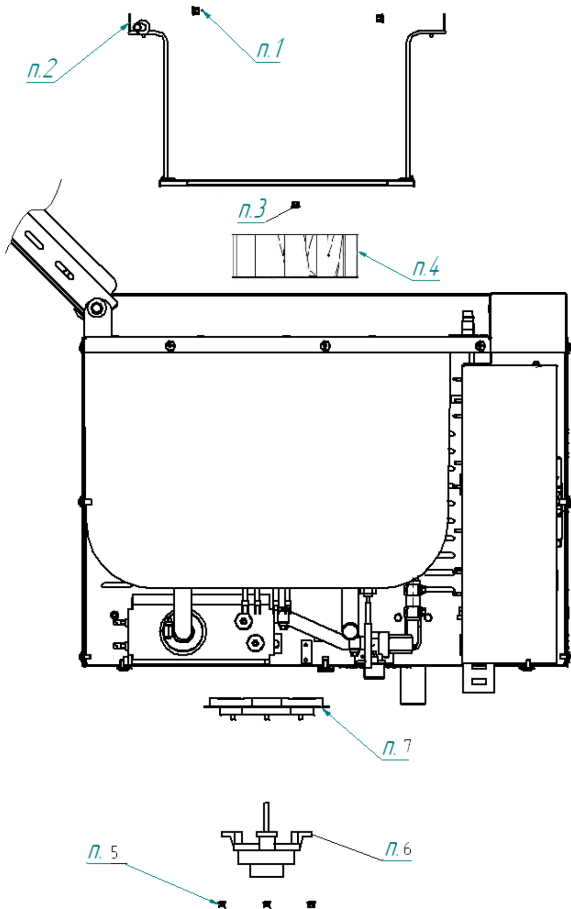
Рис. 6. Схема замены манжет
