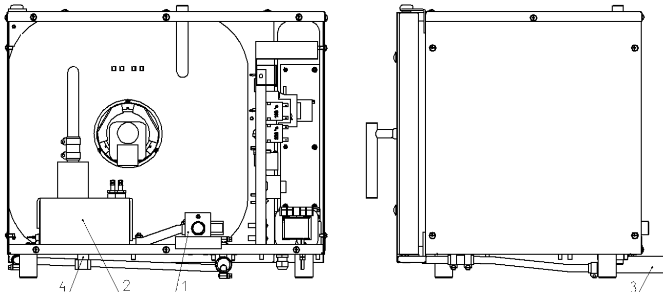
Рис. 2. Система водоснабжения и водоотведения
