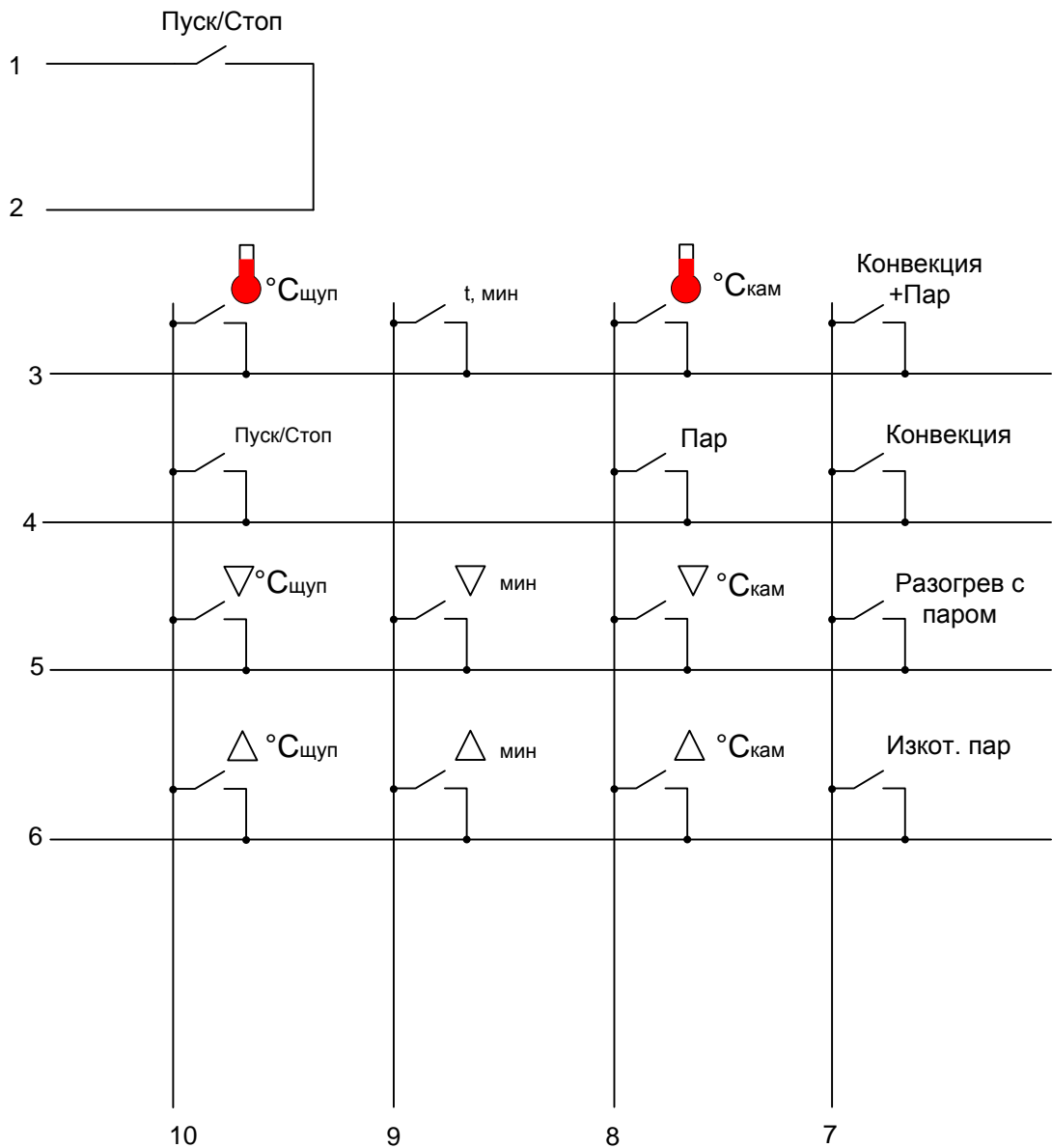
Рис. 8 Схема клавиатуры
