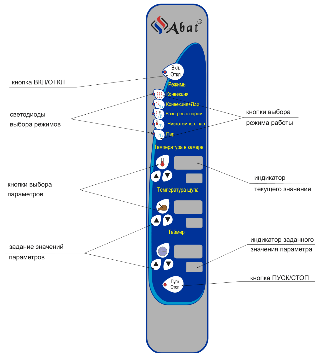
Рис. 3. Панель управления ПКА
