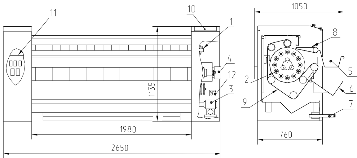
Рис.1. Общий вид
