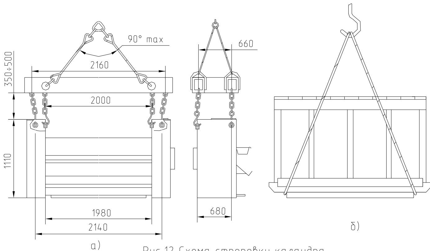
Рис.12 Схема строповки каландра а) без тары; б) в таре
