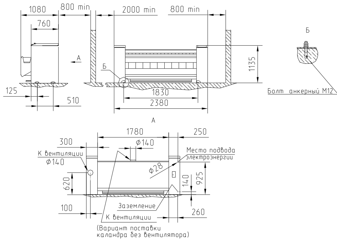
Рис.7. Монтажный чертёж
