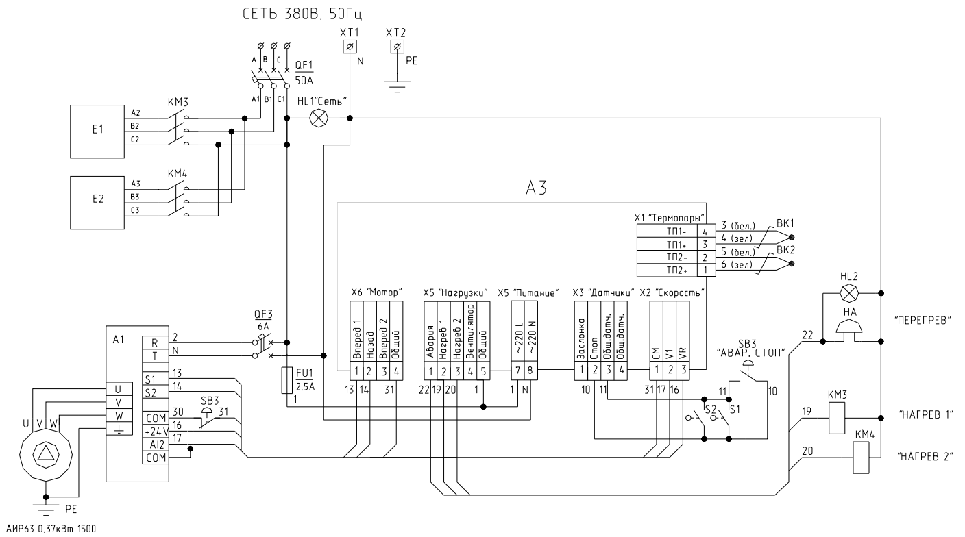
Рис. 3з. Схема электрическая принципиальная каландра гладильного ЛК1640 без вентилятора
