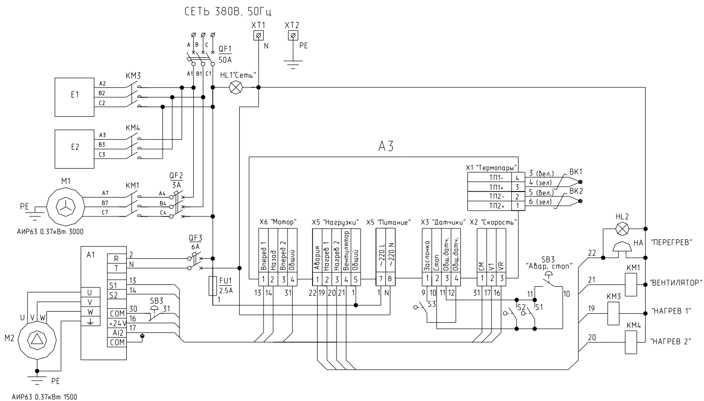
Рис. 3б. Схема электрическая принципиальная каландра гладильного ЛК1640 с вентилятором
