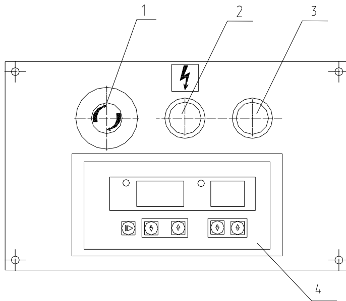
Рис. 5. Расположение органов управления каландра гладильного ЛК1840
