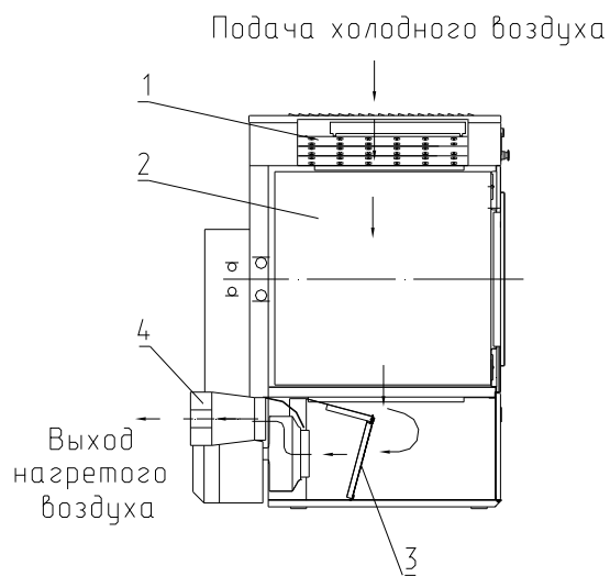
Рис.3. Схема движения воздуха.
