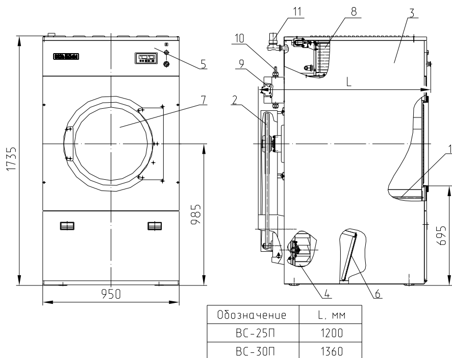
Рис.1. Общий вид
