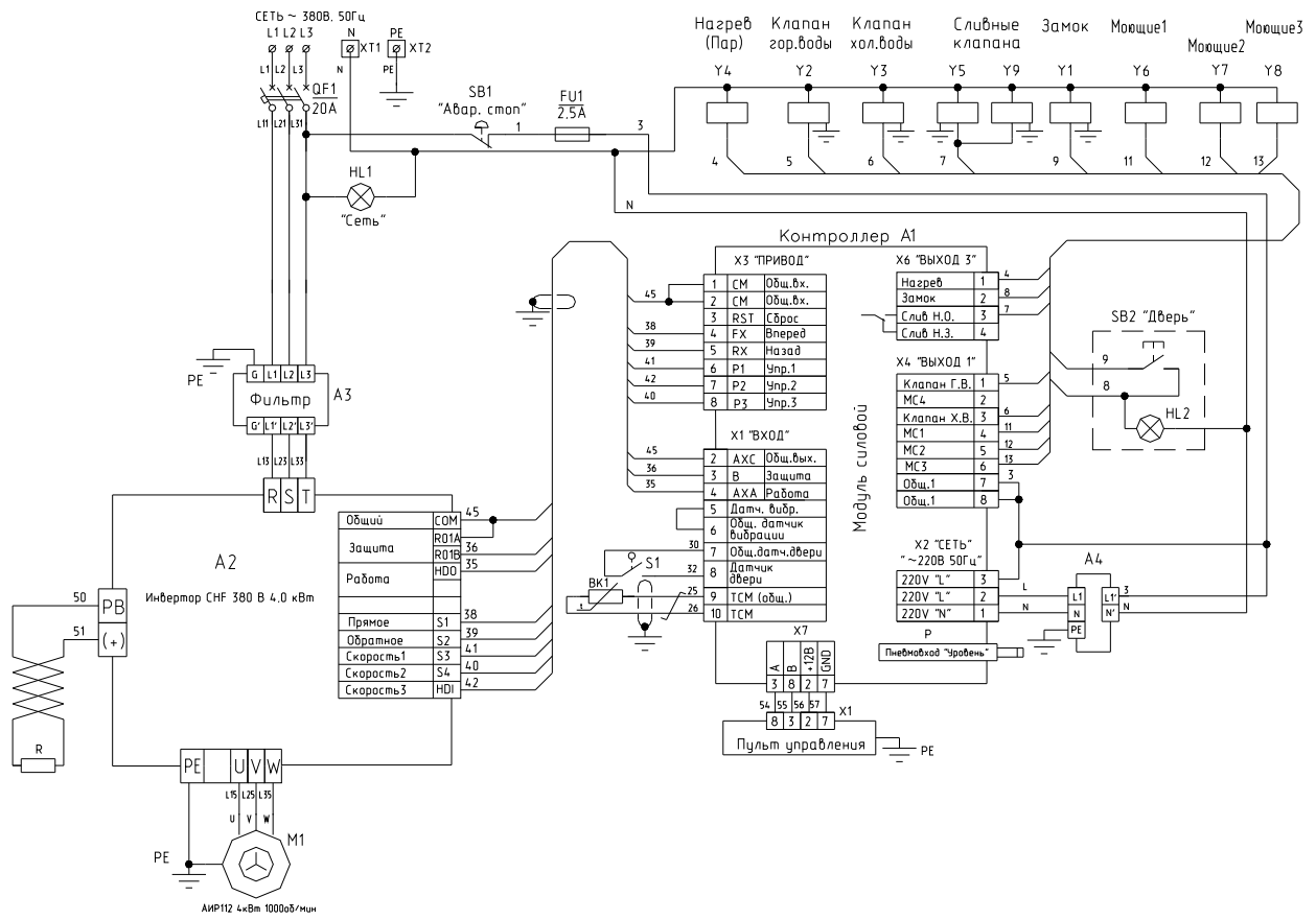
Рис.4а. Схема электрическая принципиальная машины стиральной В35-322
