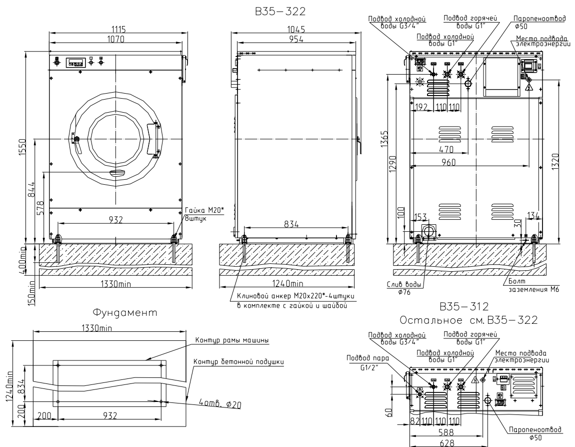
Рис.6 Монтажный чертеж
