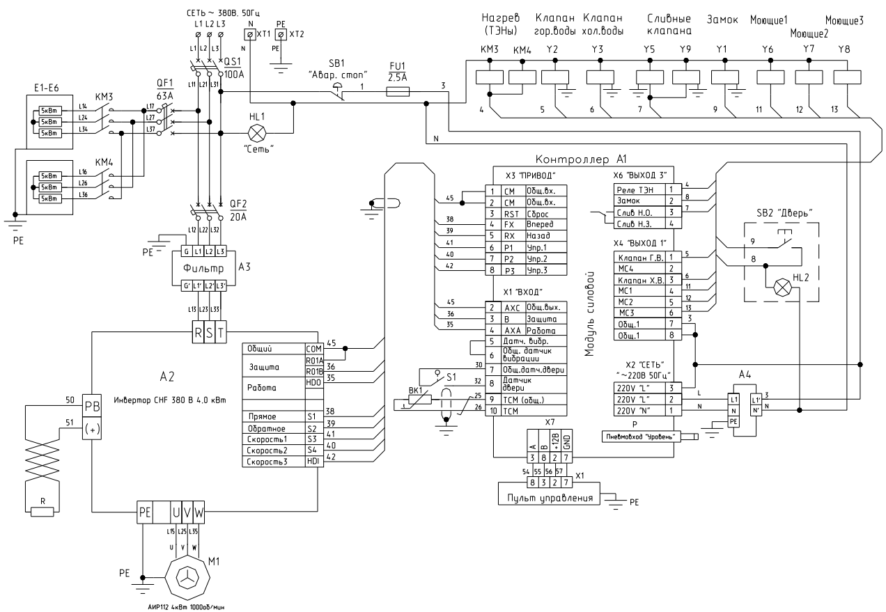
Рис.4б. Схема электрическая принципиальная машины стиральной В35-312
