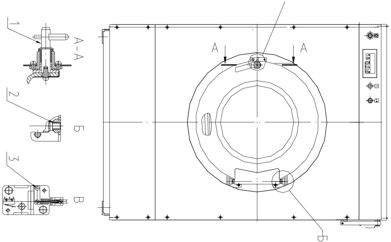
Рис.7 Схема смазки 1. Ось затвора замка. 2. Оси газоразночного люка. 3. Ось статора.
